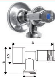
TORNEIRA ARCO L-85
