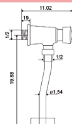
TEMPORIZADOR PARA TORNEIRA URINOL LUXO
