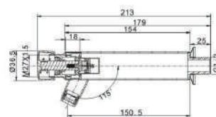
TORNEIRA TEMPORIZADA BANCA LUXO GRANDE 18CM
