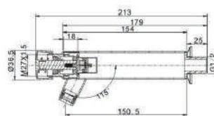
TORNEIRA TEMPORIZADA BANCA LUXO PEQUENA 14CM
