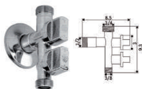
TORNEIRA ARCO DUPLA
