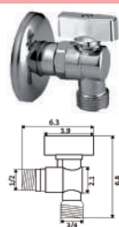
TORNEIRA CORTE MÁQUINA LAVAR TML
