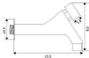
TEMPORIZADOR PARA TORNEIRA BANCA
