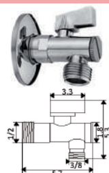
TORNEIRA CORTE COM FILTRO PEQUENA TML
