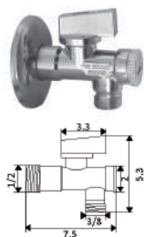
TORNEIRA ARCO MINI-FILTRO
