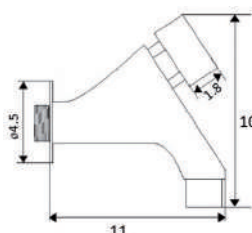
TEMPORIZADOR PARA TORNEIRA BANCA PEQUENA
