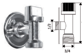
TORNEIRA ARCO L-86
