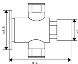
TEMPORIZADOR PARA PASSADOR EXTERIOR IDRAL
